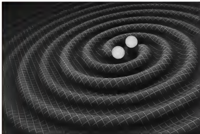
(رسم توضيحي لكيفية تكون موجات الجاذبية التي تسري في النسيج الكوني Spacetime في ضوء فرضيات النسبية ومشروع لايجو L.I.G.O)
