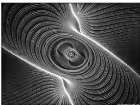
(صورتان تخيليتان لشكل الأوتار الفائقة)
