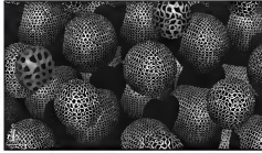
(شكل تخيلي لتكوين الذرات من الأوتار الفائقة)
