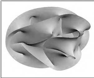
(صورتان تخيليتان لشكل الأسطح المتداخلة على بعضها في افتراضات ميكانيكا الكم)
